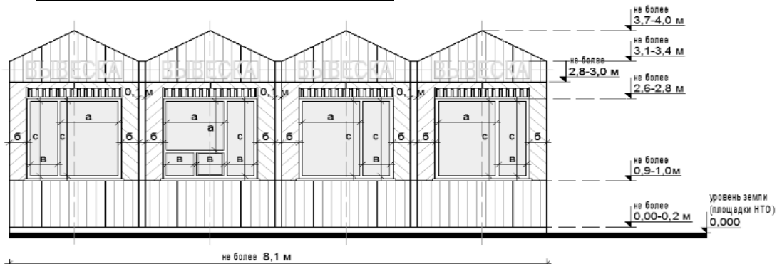
схема с максимальными размерами:
