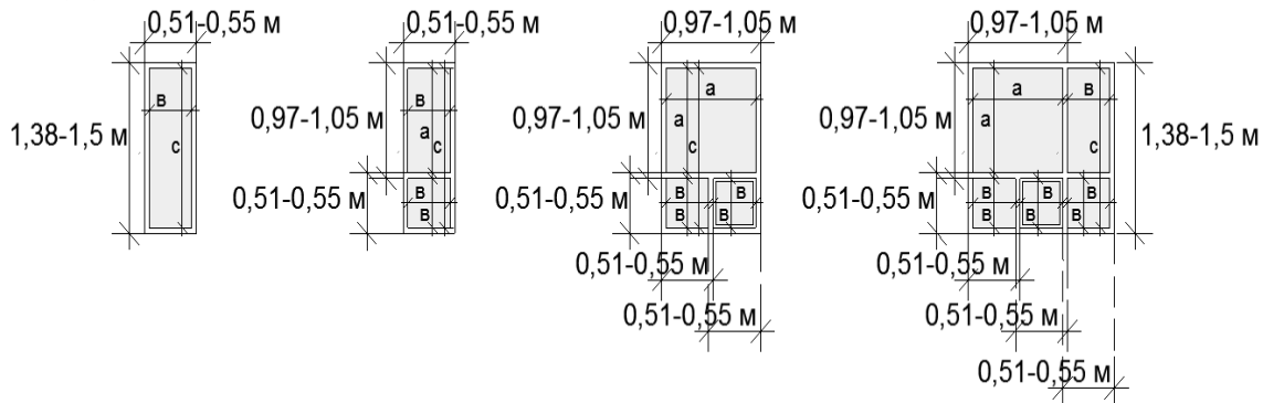
схема допустимого увеличения площади остекления:
