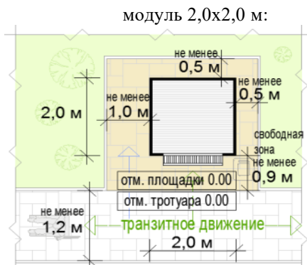
Рис. «Основные параметры места размещения нестационарного торгового объекта для палаток» схемы места размещения нестационарного торгового объекта при островном размещении модуля палатки:
