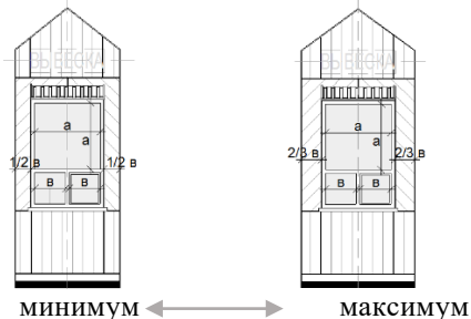
схема допустимого увеличения простенков:
