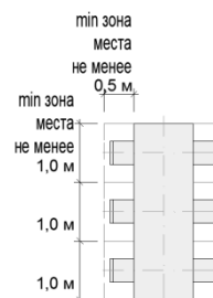
Рис. «Основные параметры расстановки мебели на площадках сезонных (летних) кафе» размещение столов и стульев:
