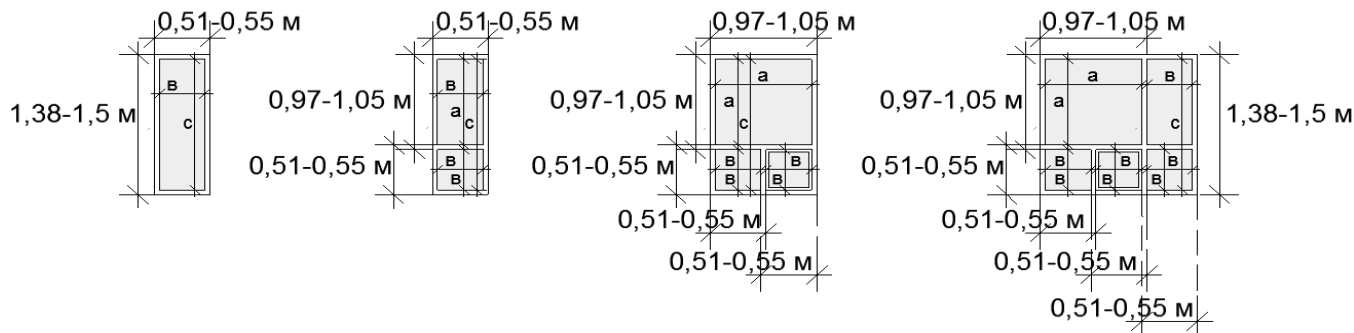
схема допустимого увеличения площади остекления:
