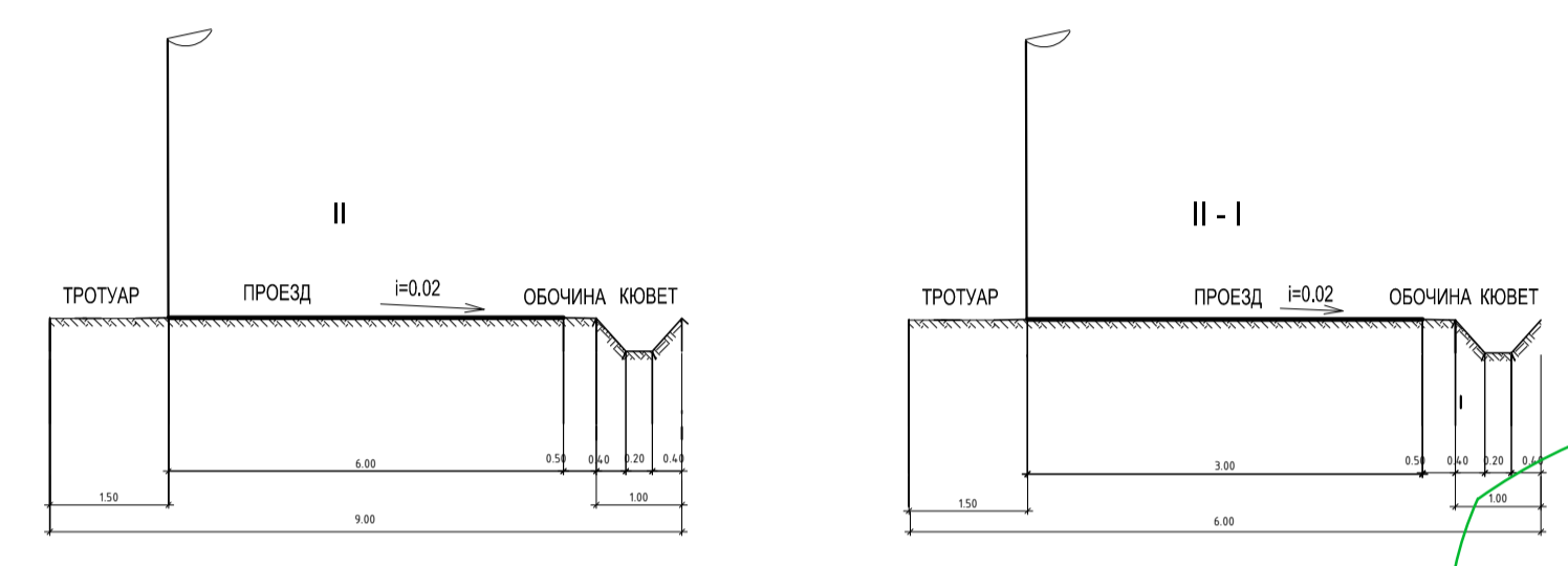
Поперечные профили дорог
