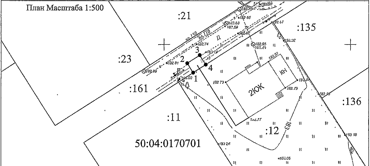
Каталог координат поворотных точек контура проектируемого сооружения
